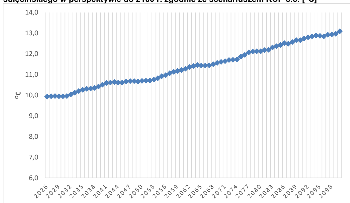
Rysunek 4 Prognozowany przyrost średniej rocznej temperatury powietrza na terenie powiatu sulcińskiego w perspektywie do 2100 r. zgodnie ze scenariuszem RCP 8.5. [°C]
